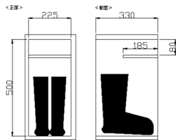
<ロッカー内寸図>
